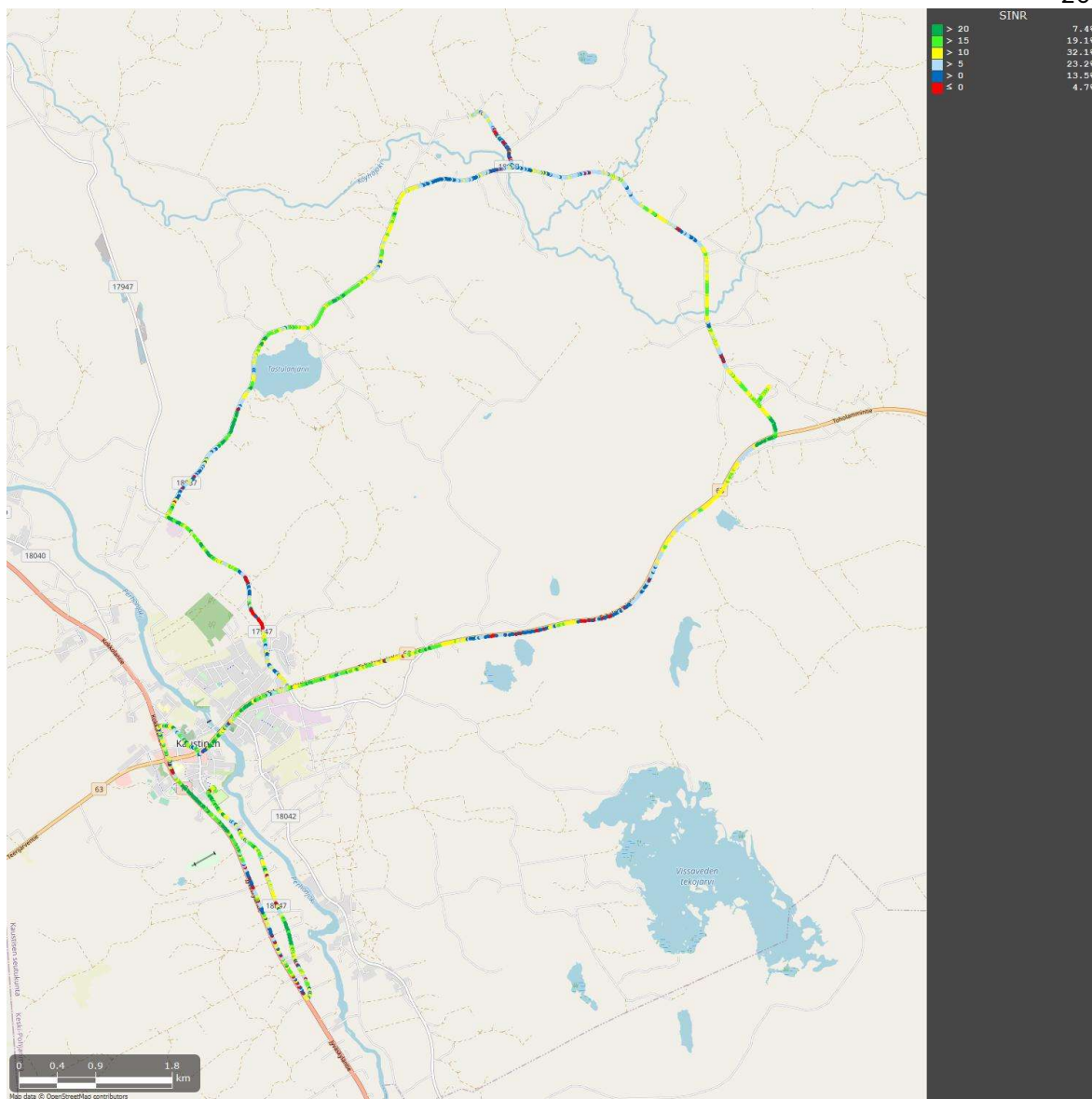
4G: SINR
