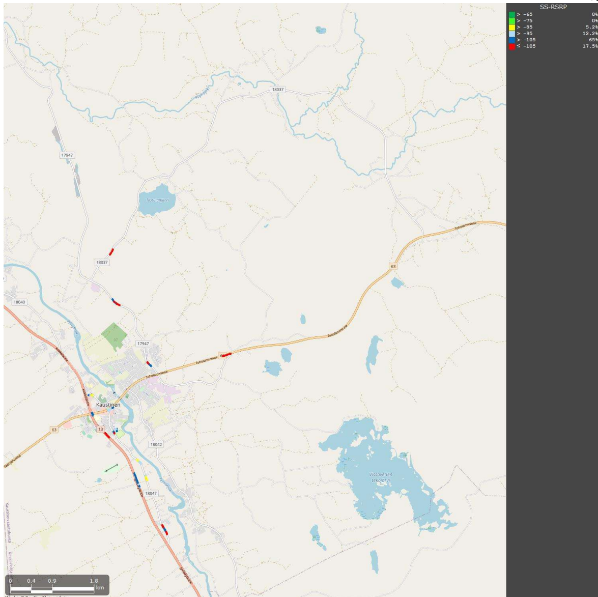
5G: SS-RSRP
